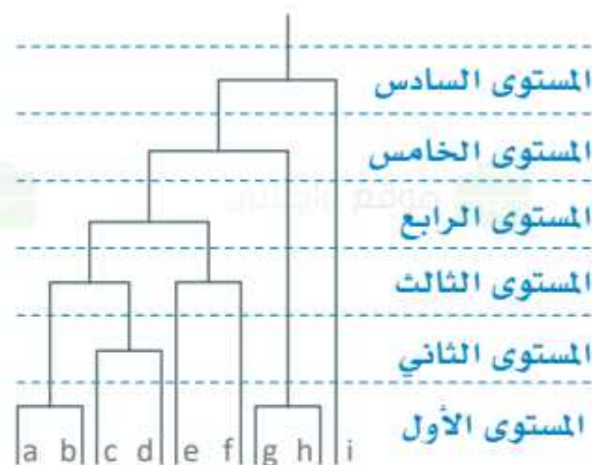
شكل 3.19: التجميع التكتلي (AC)
