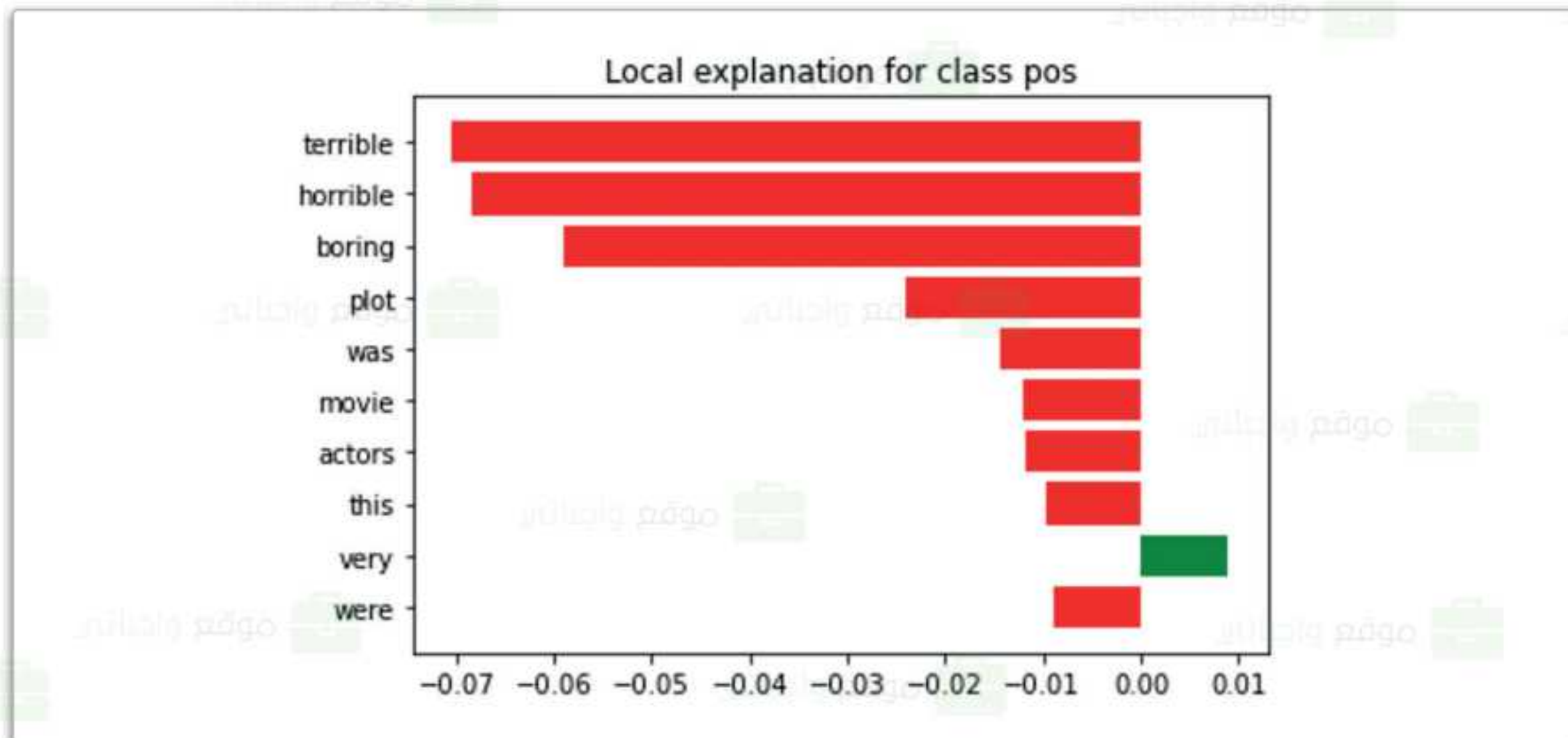
شكل 3.9: الكلمات الأعلى تأثيراً في القيام بالتنبؤات
