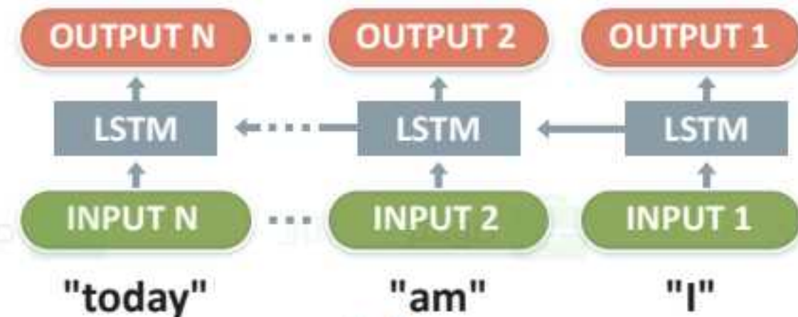
شكل 3.29: الذاكرة المُطوِّلة قصيرة المدى
